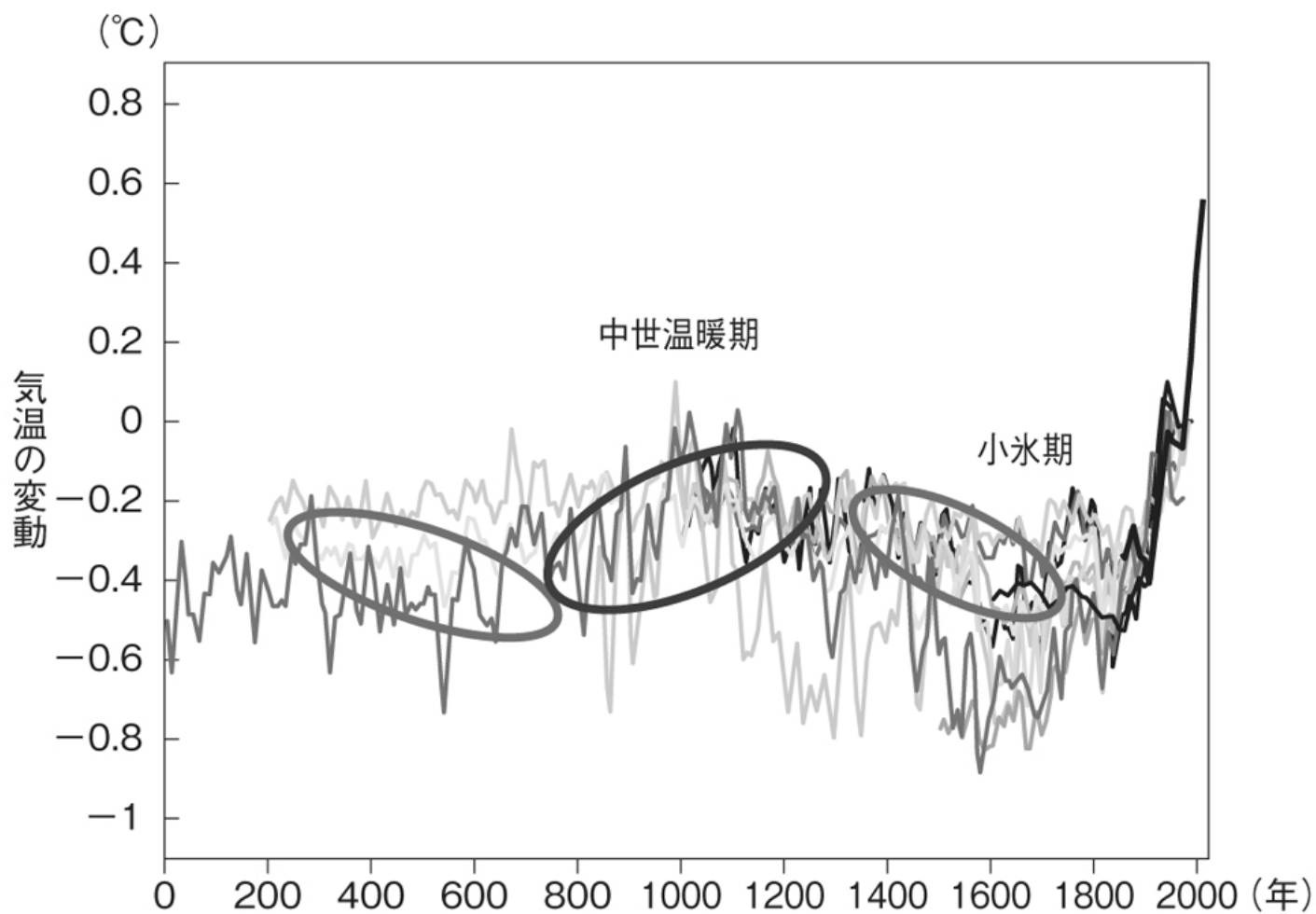
図表2-1 北半球の気温変動
